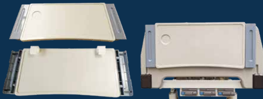
AB-02-1 ABS塑鋼/聚酯伸縮餐桌板 (掛勾: 塑膠or橡膠 / 不超出床體寬度 )
